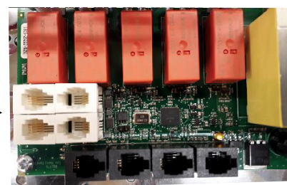
Imagen 5. Orden de los conectores RJ 10. Sensor, interruptor de puerta, control remoto, NTC adicional
