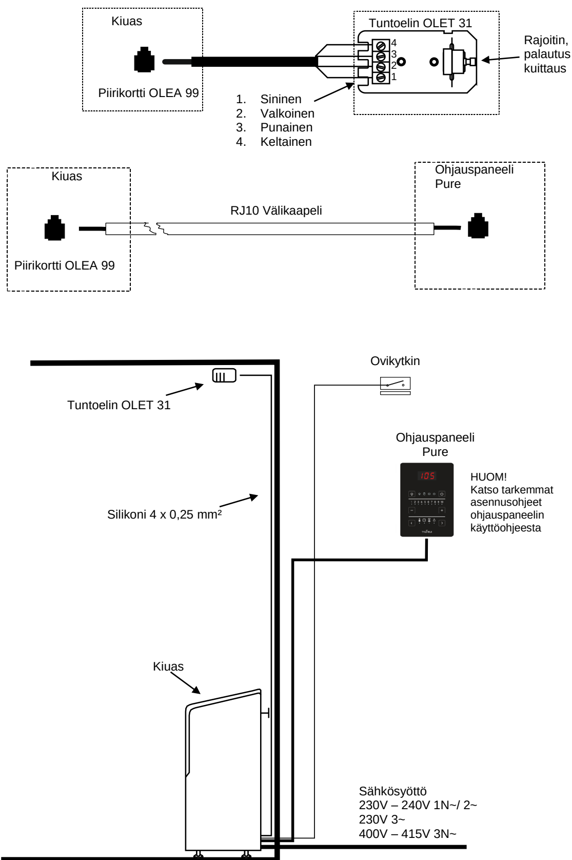
Kuva 9 Periaatekuva asennuksesta
