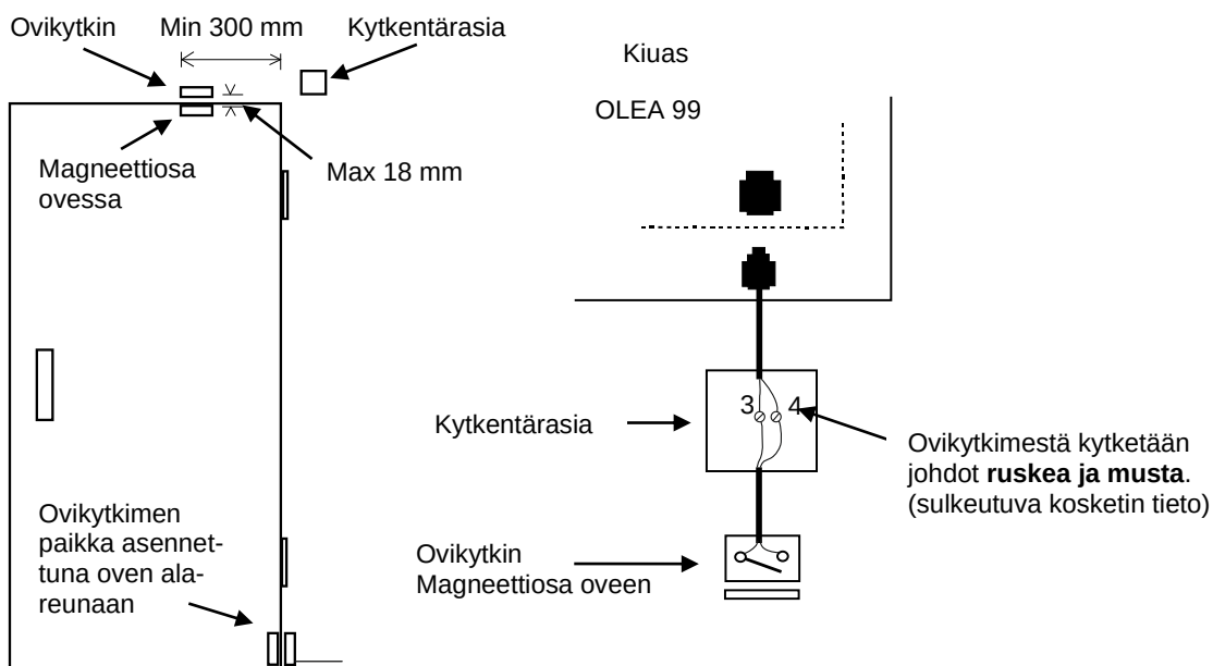
Kuva 7 Ovikyttime asento
