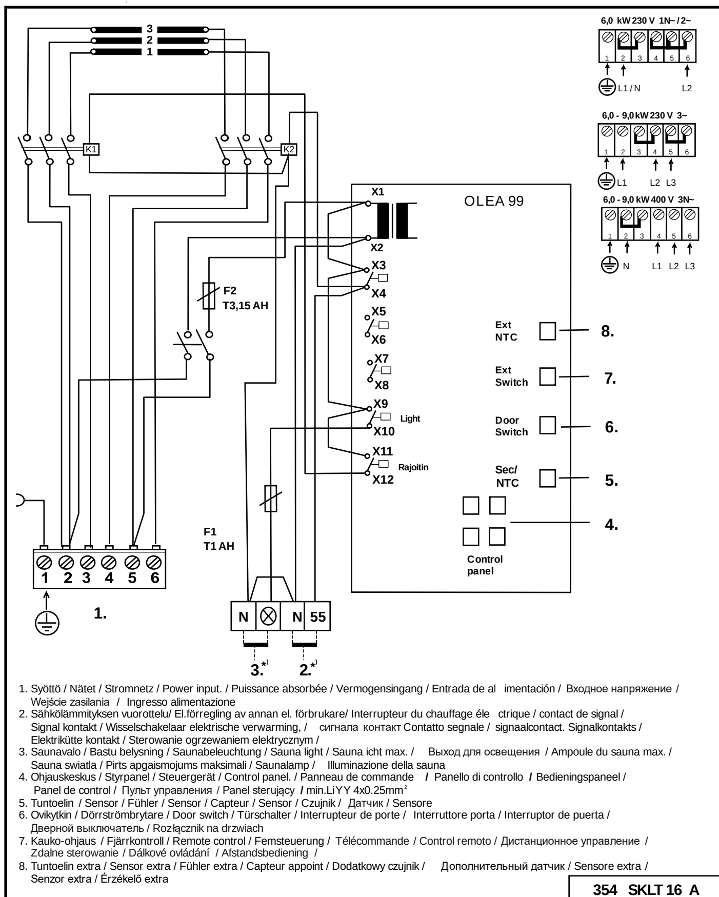
Imagen 6. Diagrama de conexiones
