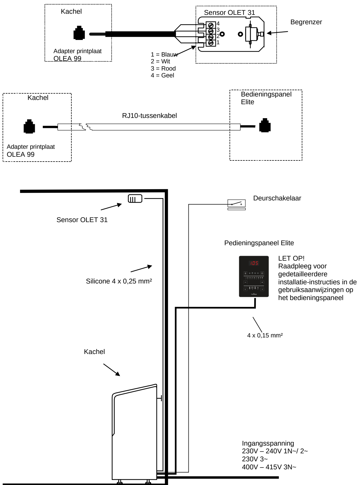
Afbeelding 9 Principe-afbeelding
