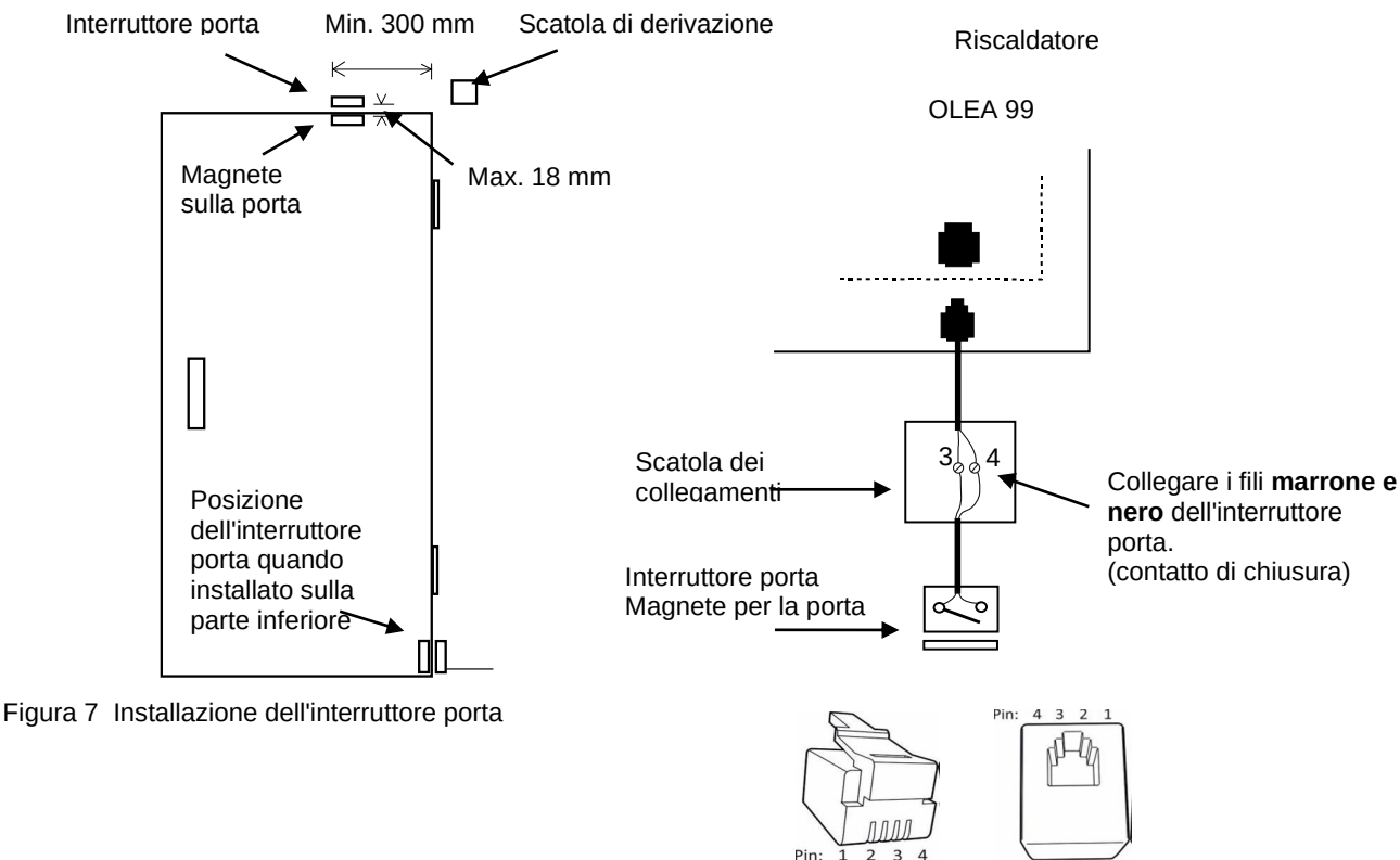
Figura 8. Pin: ordine di RJ 10
