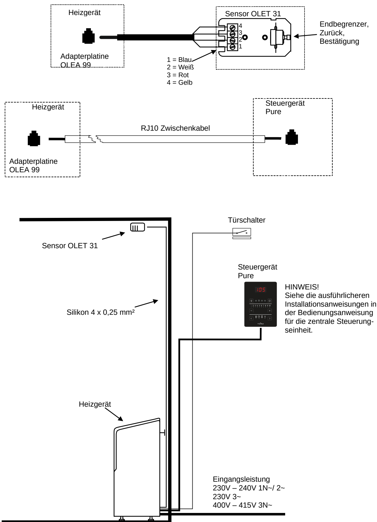
Abbildung 9 Prinzipbild
