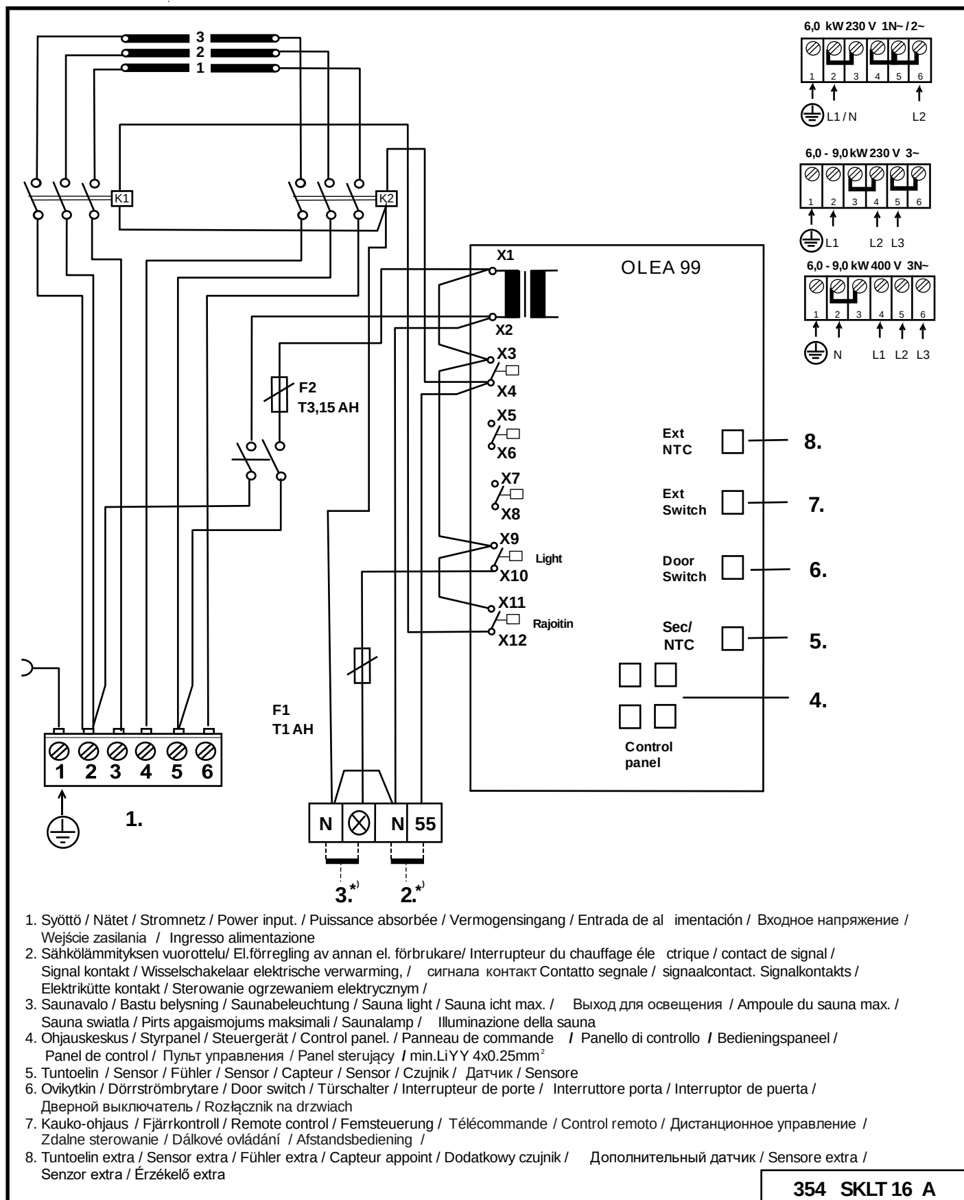
Afbeelding 6. Bedradingsschema voor de saunakachel
