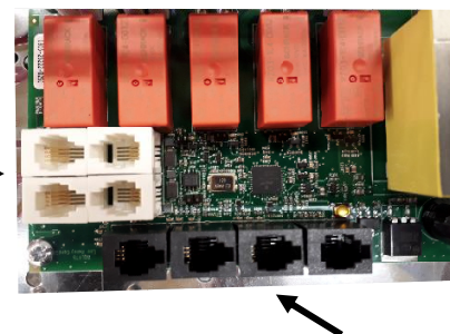
Рис 5 Расположение разъемов RJ 10. Датчик, дверной выключатель, дистанционное управление, дополнительный датчик NTC
