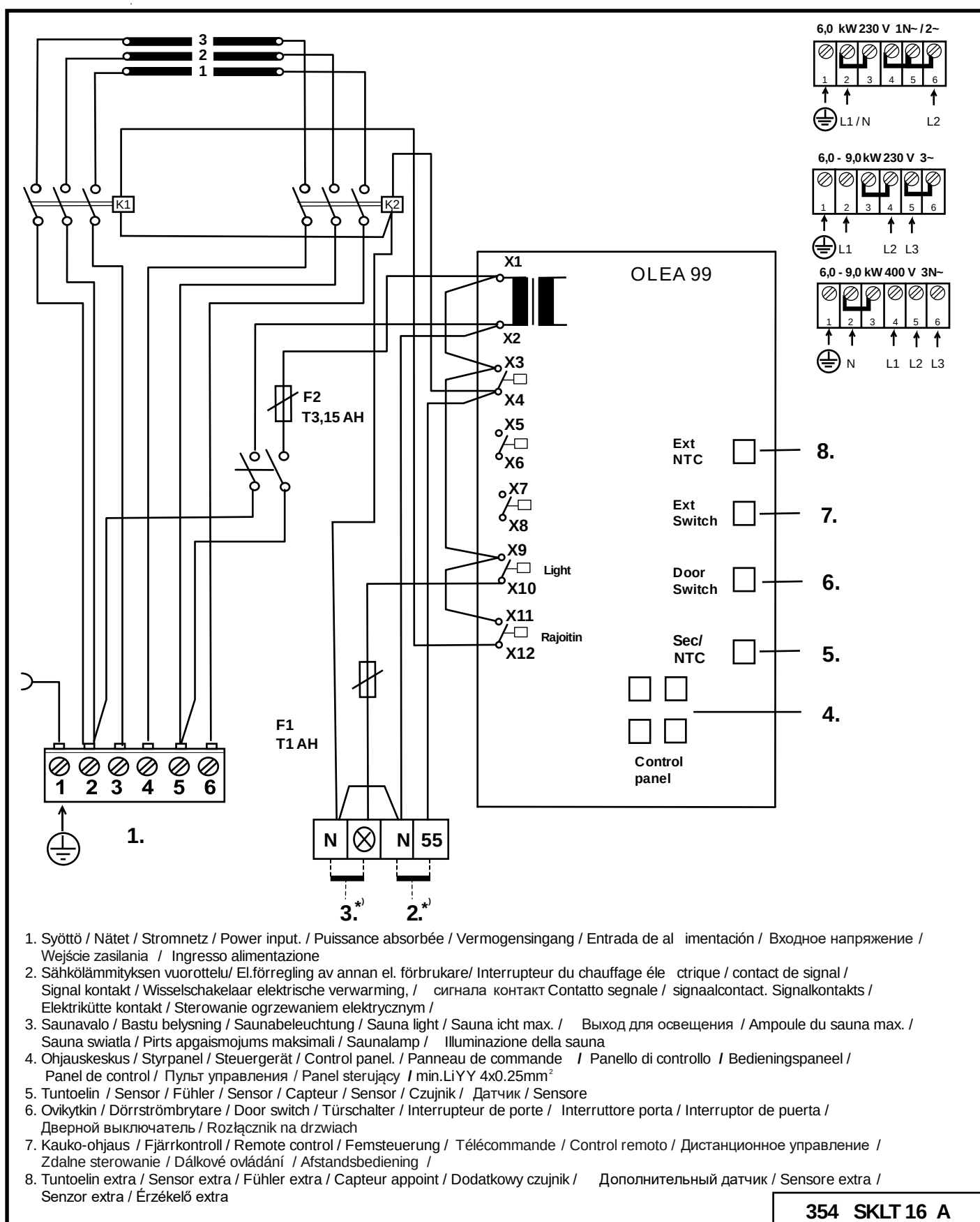
Abbildung 6. Schaltdiagramm
