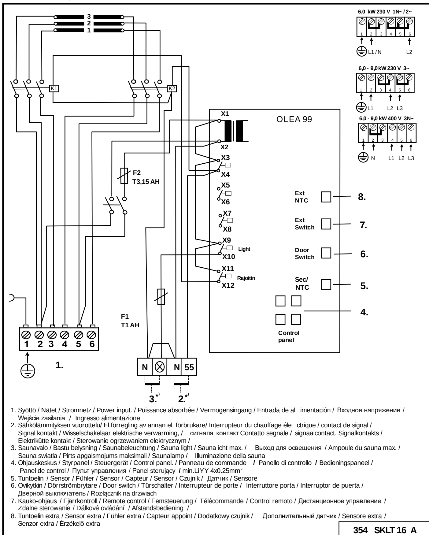
Rysunek 6. Schemat podłączenia pieca
